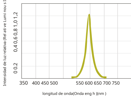
Curva característica de distribución espectral Distribución espectral relativa
