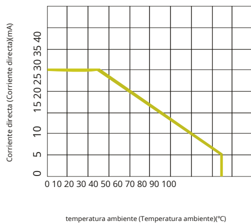
Curva de reducción de corriente directa Curva de reducción de corriente directa
