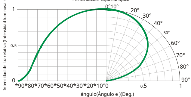
Curva característica de distribución de intensidad luminosa. Perturbación espacial típica
