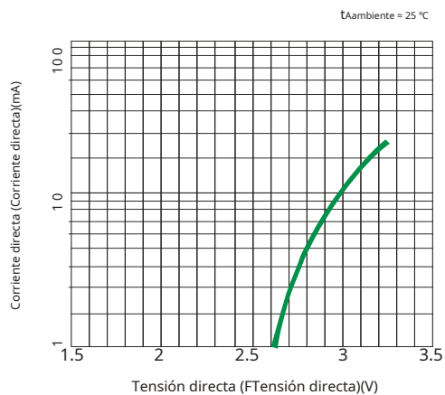
Características del voltamperio Características de voltios*amperios
