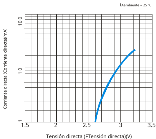
Características del voltamperio Características de voltios-amperios
