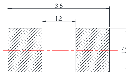
Tamaño de almohadilla recomendado Almohadilla de soldadura recomendada
