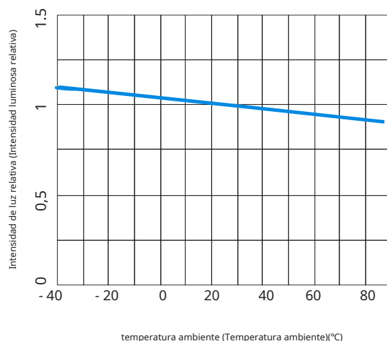
Curva de intensidad de luz y temperatura ambiente. Intensidad luminosa versus temperatura ambiente
